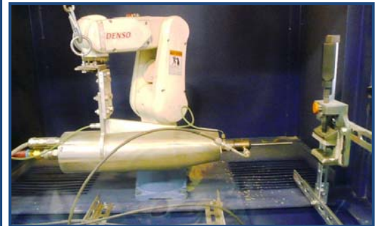
スプレーブース内 ACGS ガンヘッド
